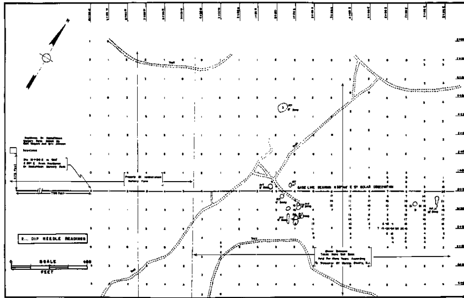
FIGURE 33 , SECTION I, SEARLE MINE , WARREN CO., N. J.
